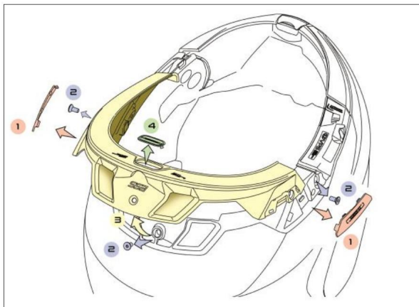
Rys. 4C – TYLKO DLA HEŁMÓW N100-6, N120-1
